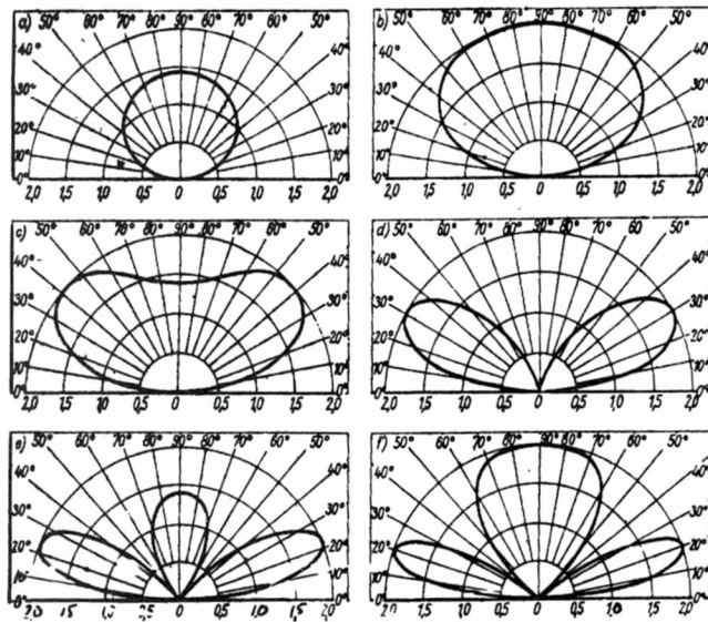
FIG. 6. Verticale stralingspatronen van horizontaal opgehangen dipolen op verschillende hoogten boven de grond. a) \frac{1}{4} golf hoog; b) \frac{1}{4} golf hoog; c) \frac{3}{8} golf hoog; d) \frac{1}{2} golf hoog; e) \frac{5}{8} golf hoog; f) \frac{3}{4} golf hoog
